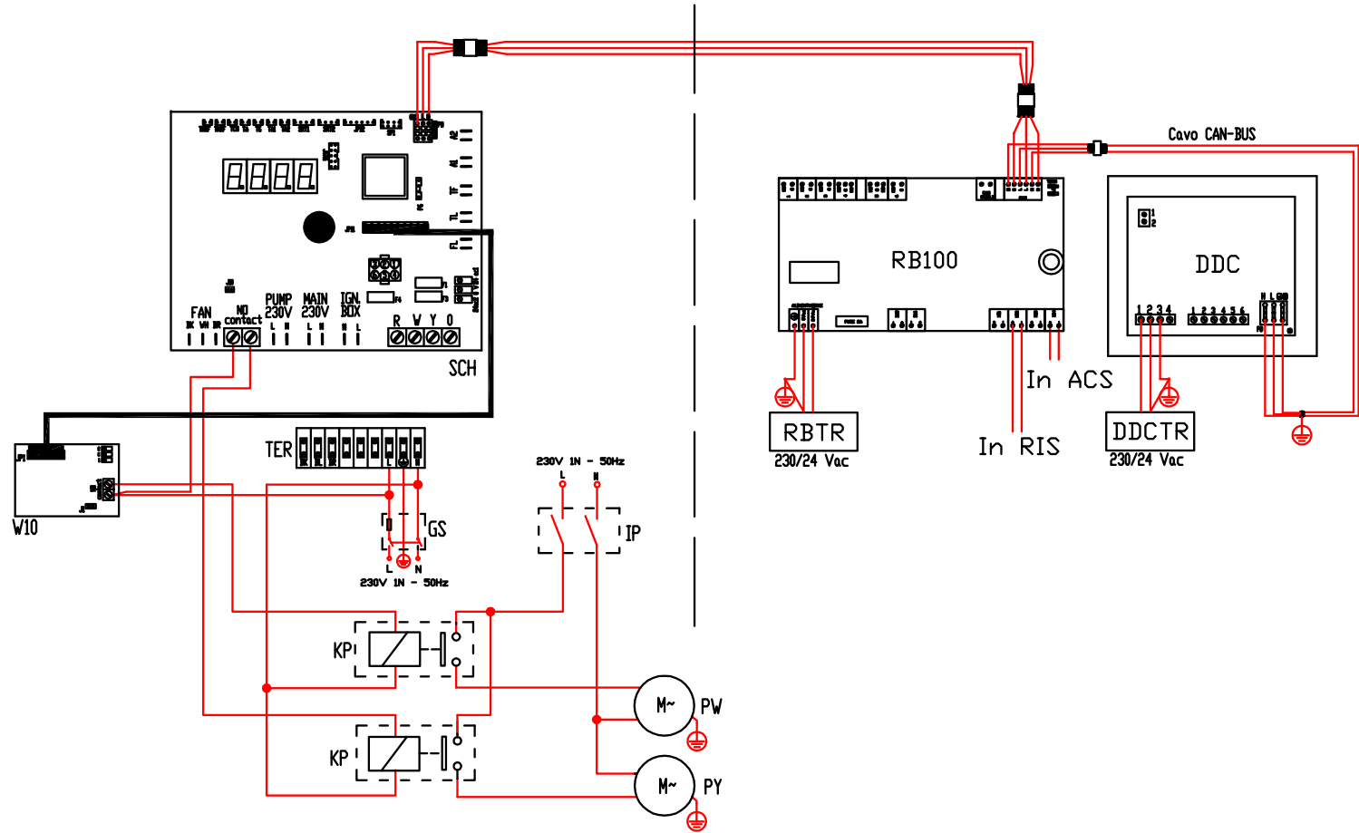
Abbildung 7.22 – Elektrische Anlage
