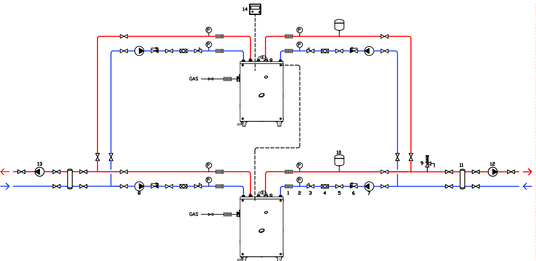
Abbildung 7.3 – Hydraulischschaltplan
