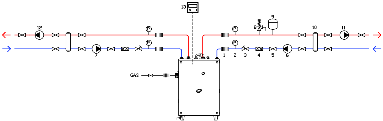
Abbildung 7.1 – Hydraulikschaltplan
