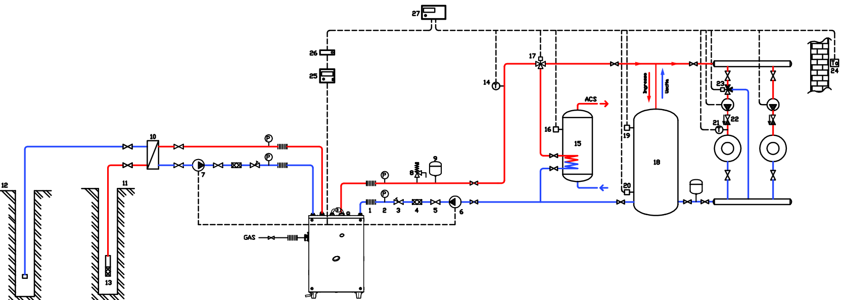
Abbildung 7.21 – Hydraulikschaltplan
