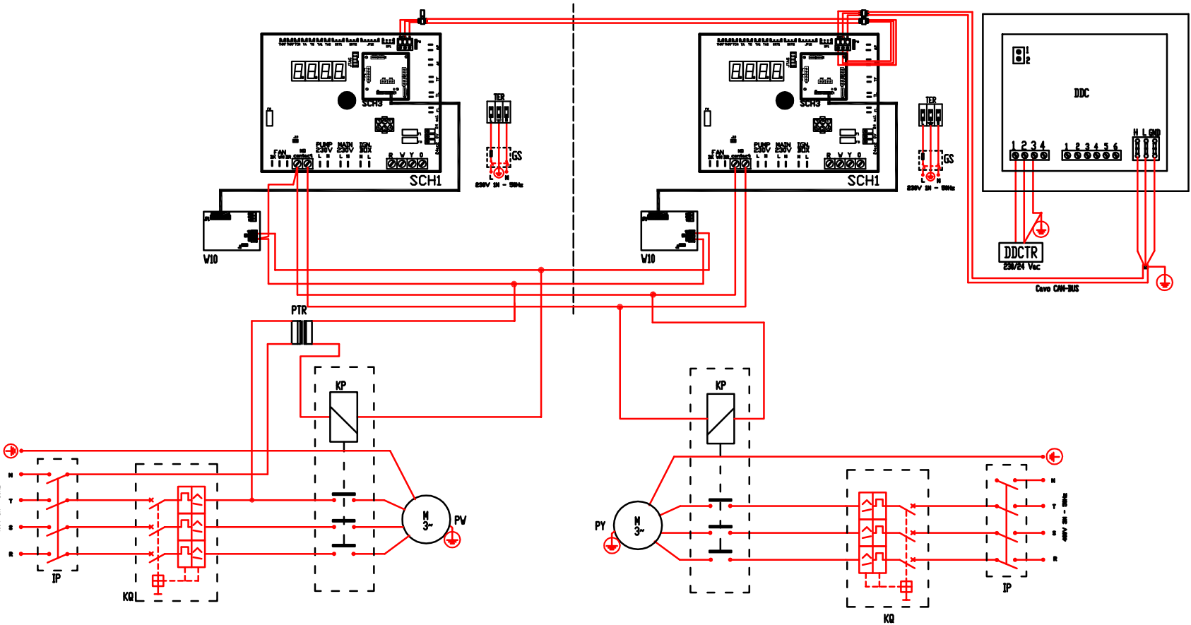
Abbildung 7.16 – Elektrische Anlage
