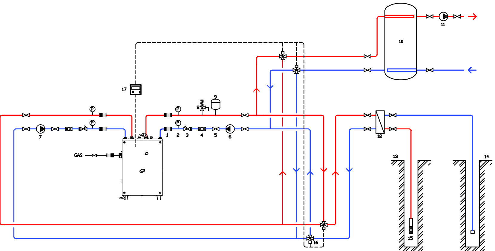
Abbildung 7.11 – Hydraulischschaltplan
