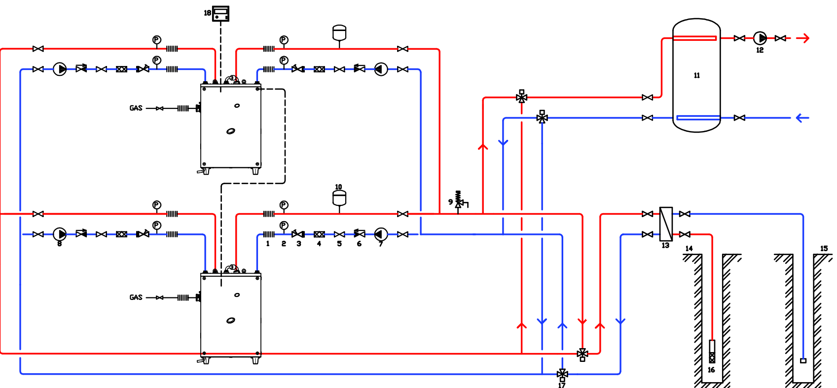
Abbildung 7.13 – Hydraulischschaltplan
