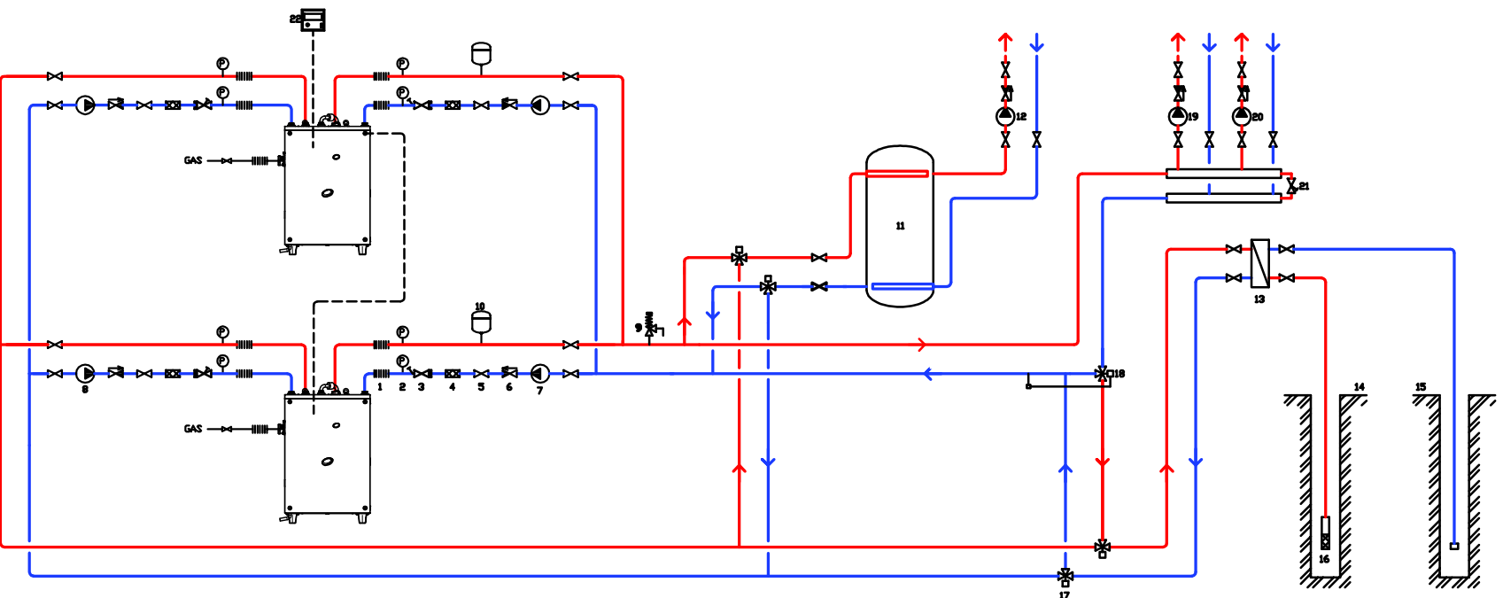
Abbildung 7.19 – Hydraulikschaltplan
