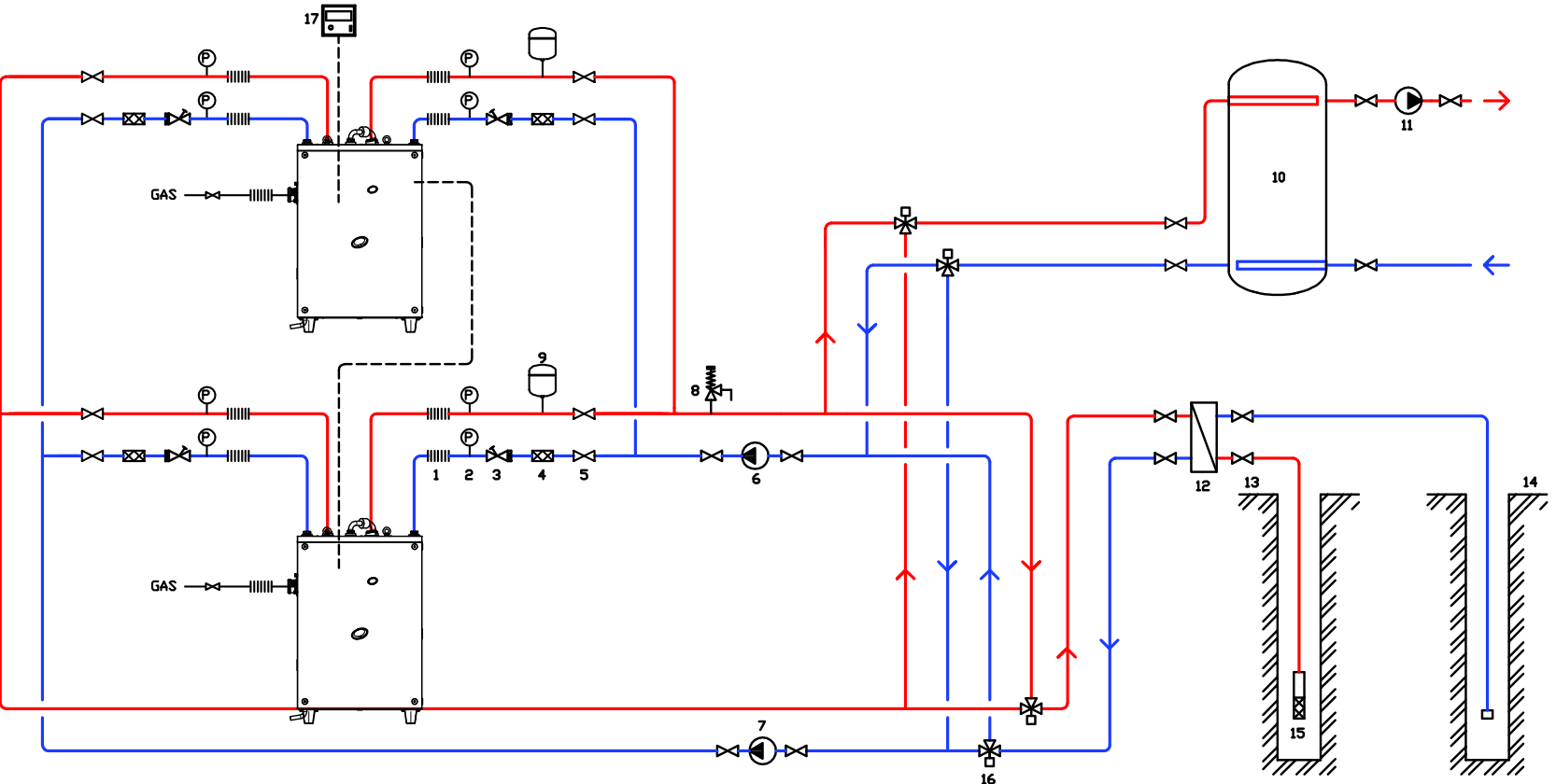
Abbildung 7.15 – Hydraulikschaltplan
