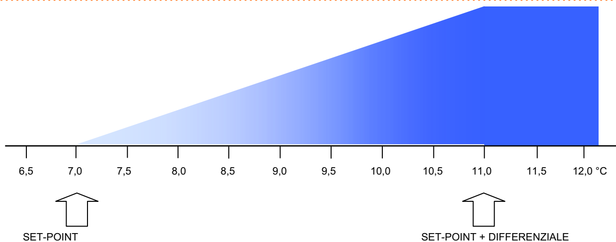
Abbildung 6.3 – Beispiel des Teillastbetriebs der Einheiten im Sommer
