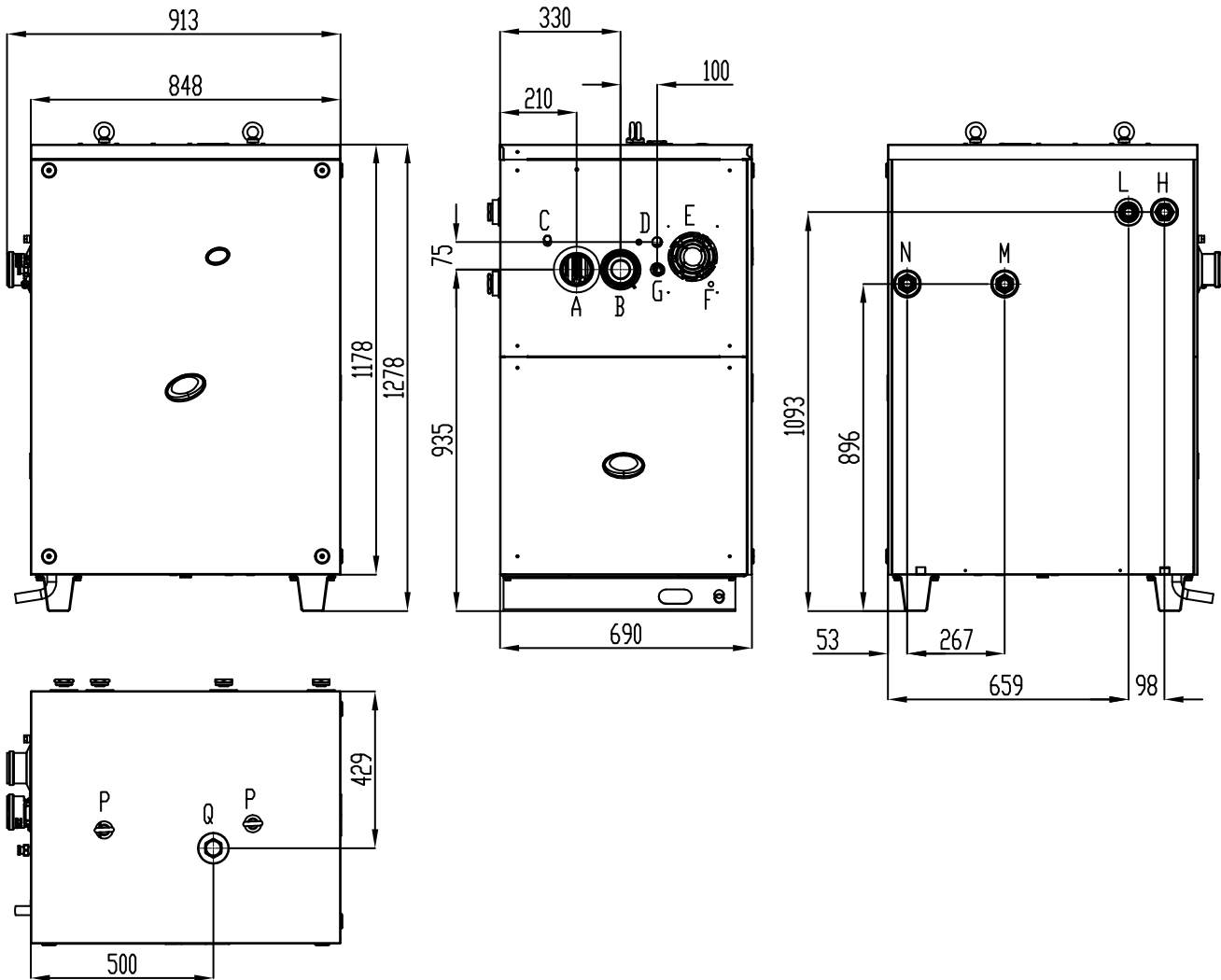
Abbildung 1.1 – Abmessungen
