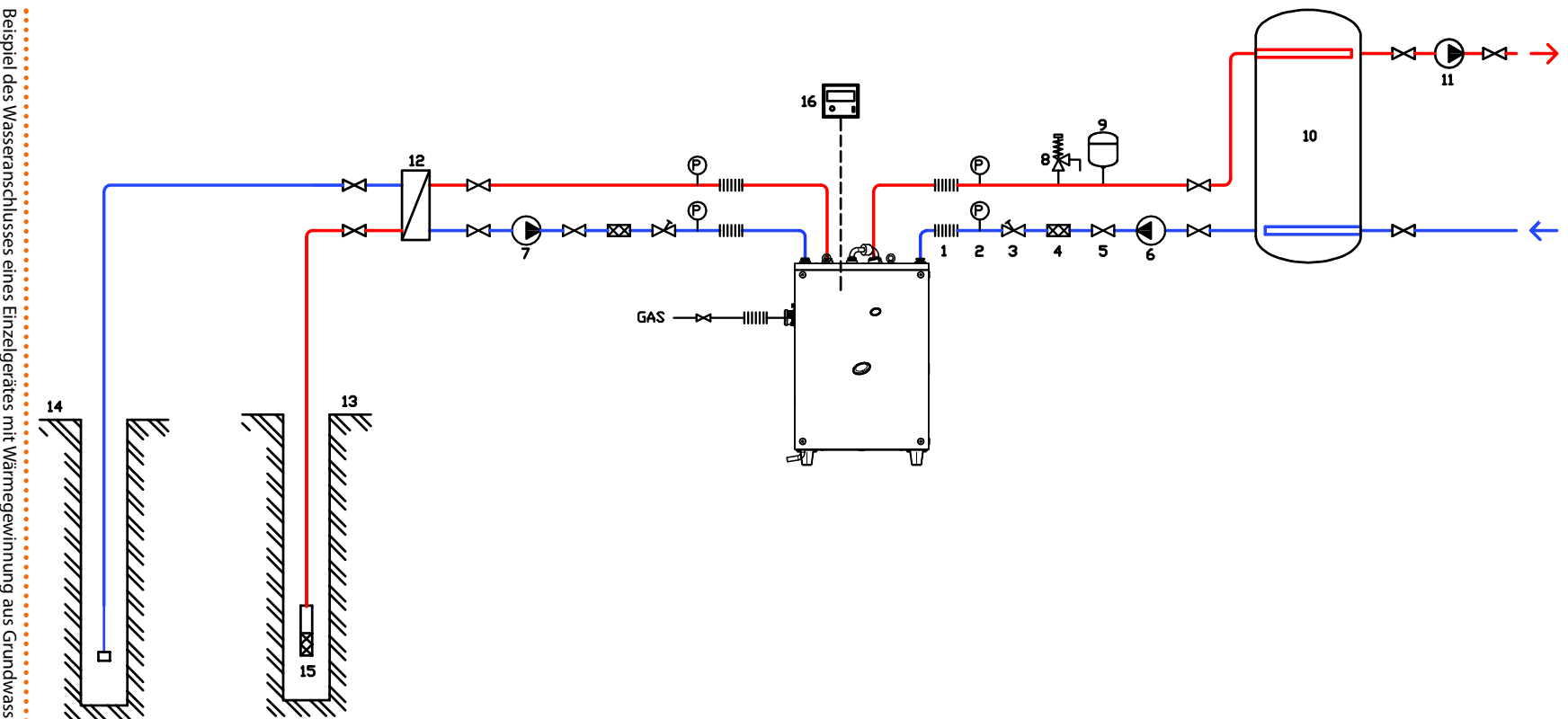
Abbildung 7.5 – Hydraulischschemaplan
