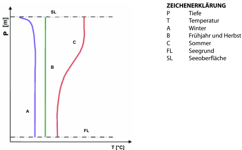
Abbildung 3.4 – Temperaturprofile in einem See
