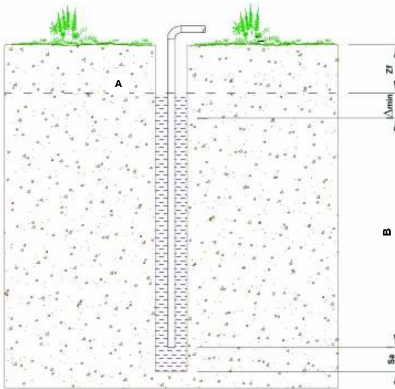
Abbildung 3.3 – Schluckbrunnen im freien Grundwasser
