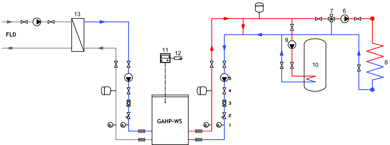
Abbildung 4.1 – Nutzung einer einzigen Einheit
