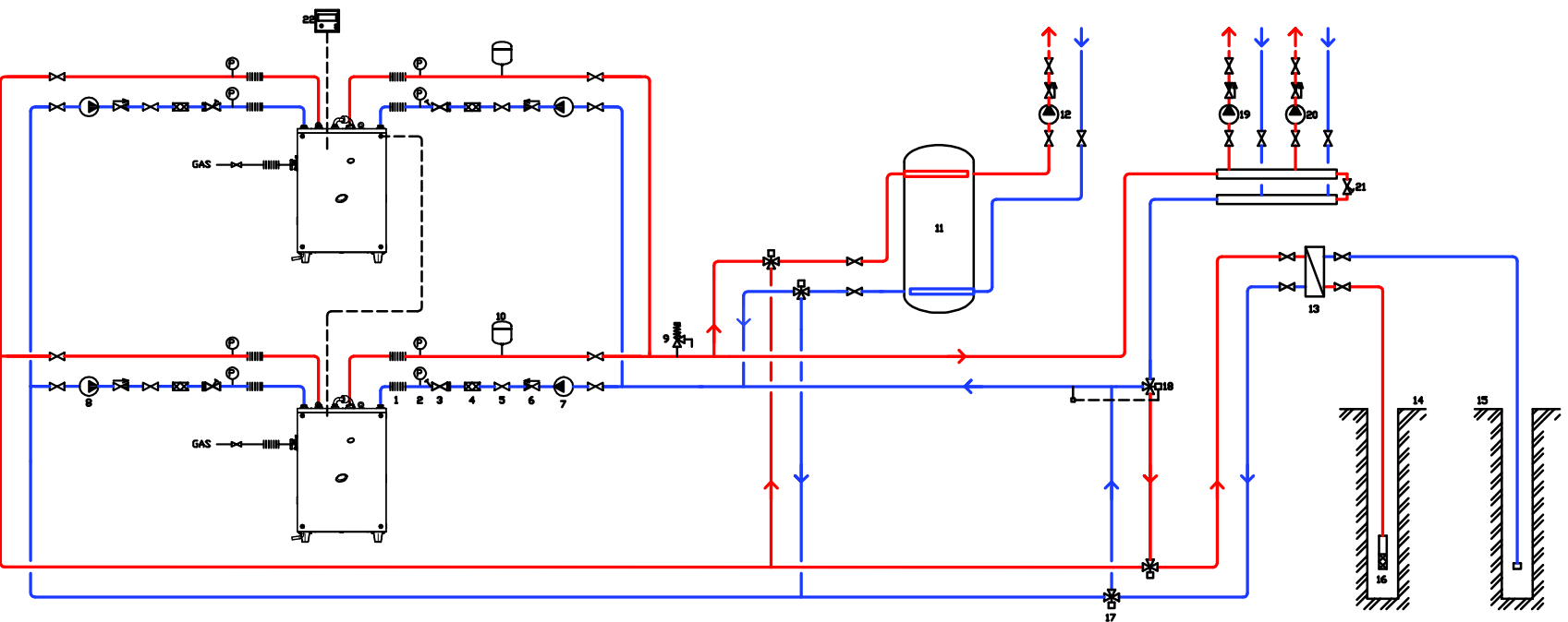
Abbildung 7.17 – Hydraulischschaltplan
