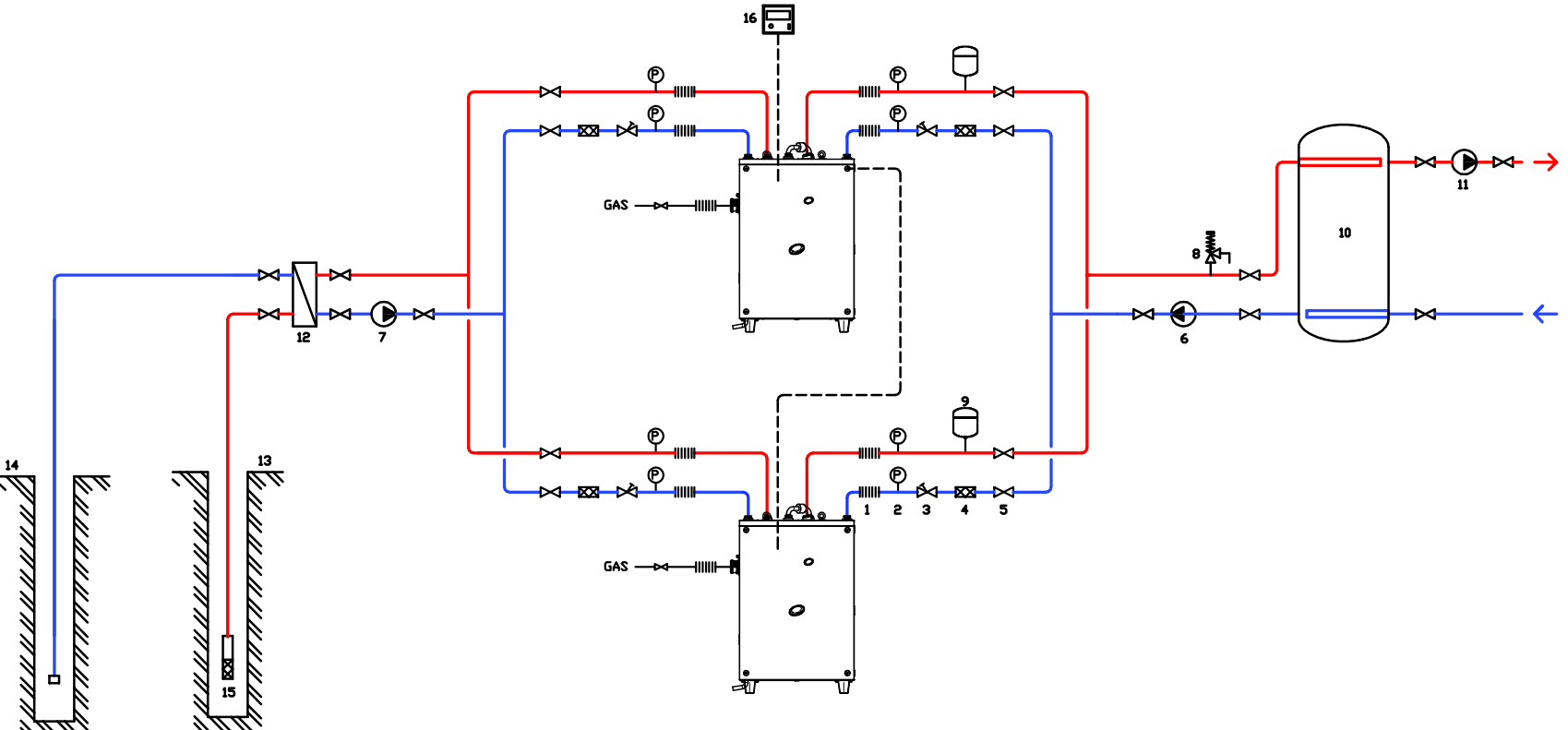
Abbildung 7.9 – Hydraulischplan
