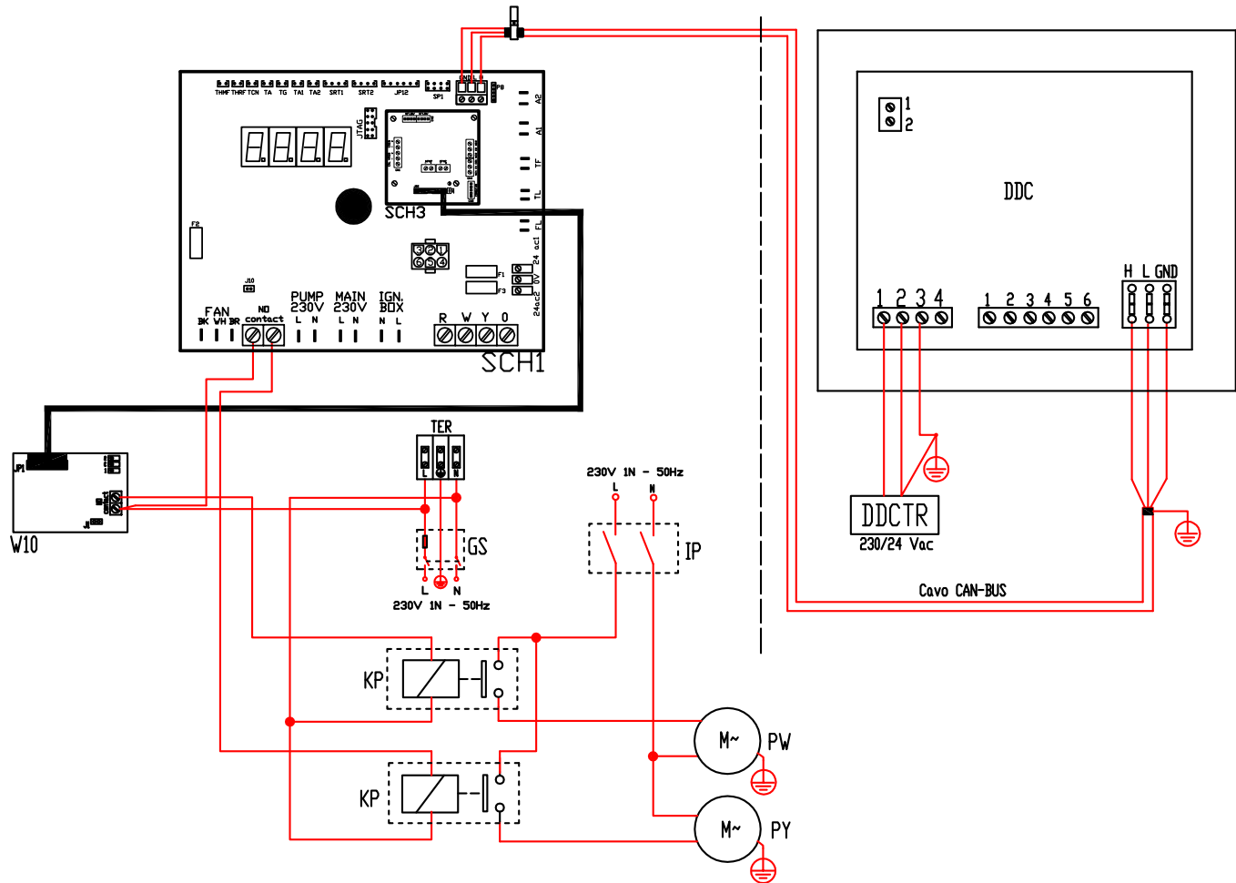
Abbildung 7.2 – Elektrische Anlage
