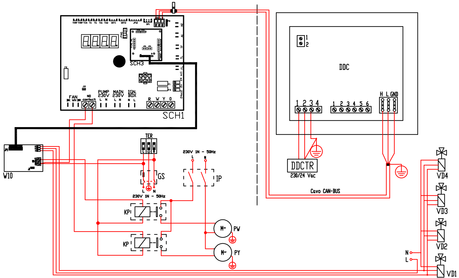
Abbildung 7.12 – Elektrische Anlage
