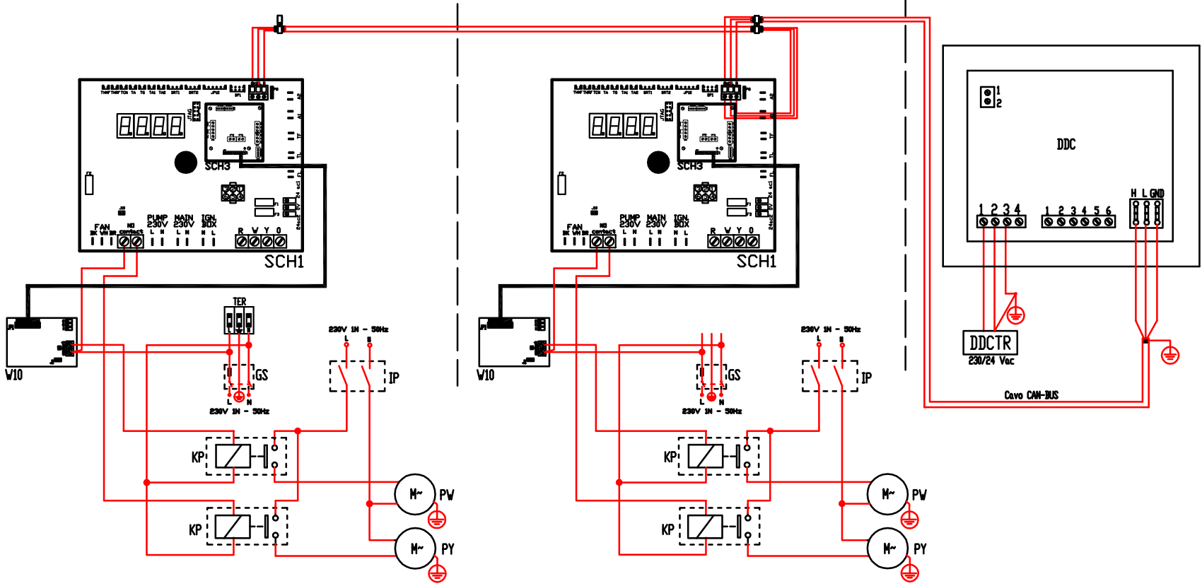
Abbildung 7.20 – Elektrische Anlage
