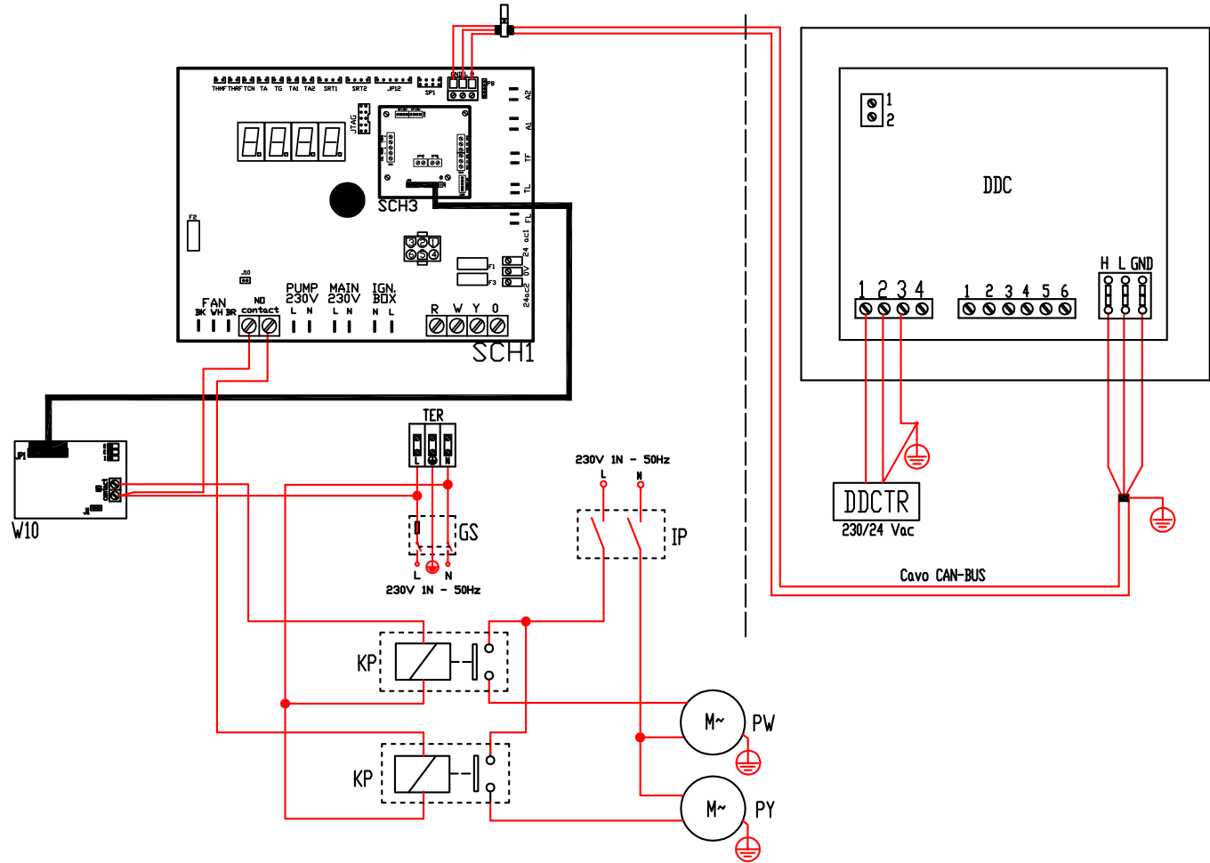
Abbildung 7.6 – Elektrische Anlage
