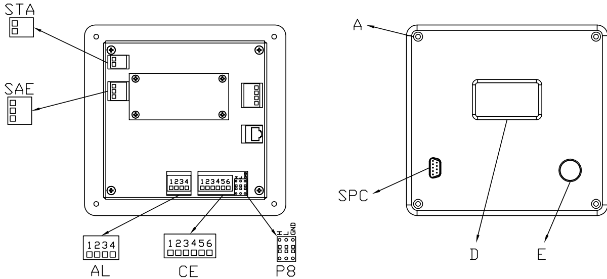
Abbildung 6.1 – Digitale Steuertafel (DDC)
