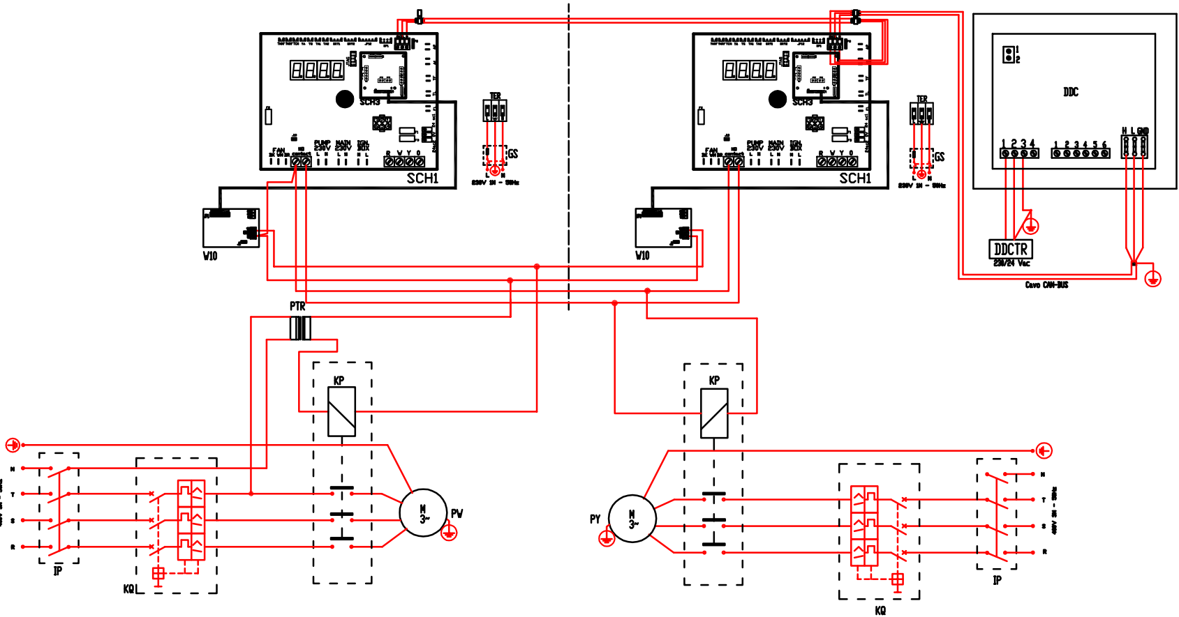
Abbildung 7.10 – Elektrische Anlage
