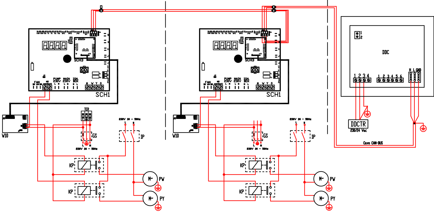
Abbildung 7.14 – Elektrische Anlage
