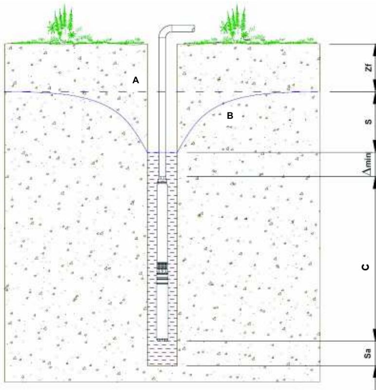
Abbildung 3.2 – Grundwasserförderbrunnen
