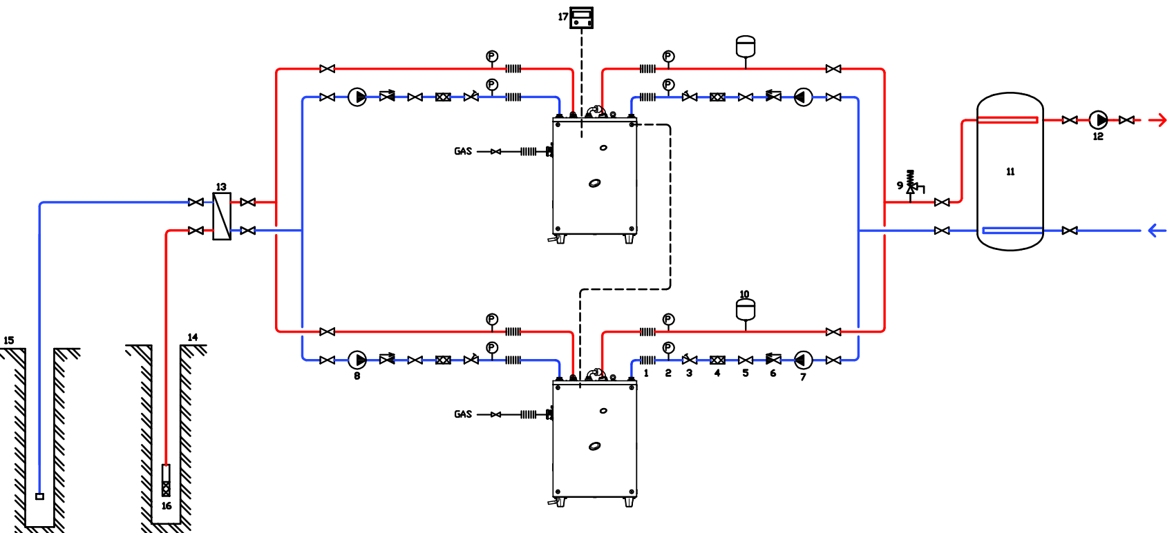
Abbildung 7-7 – Hydraulischschaltplan
