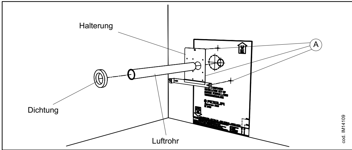
Abb. 7 BEFESTIGUNG DER HALTERUNG UND BOHRUNGEN FÜR DIE MODELLE 3001 U. 3002
