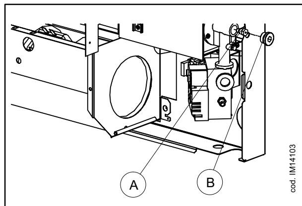
Abb. 29 BRENNERGRUPPE
