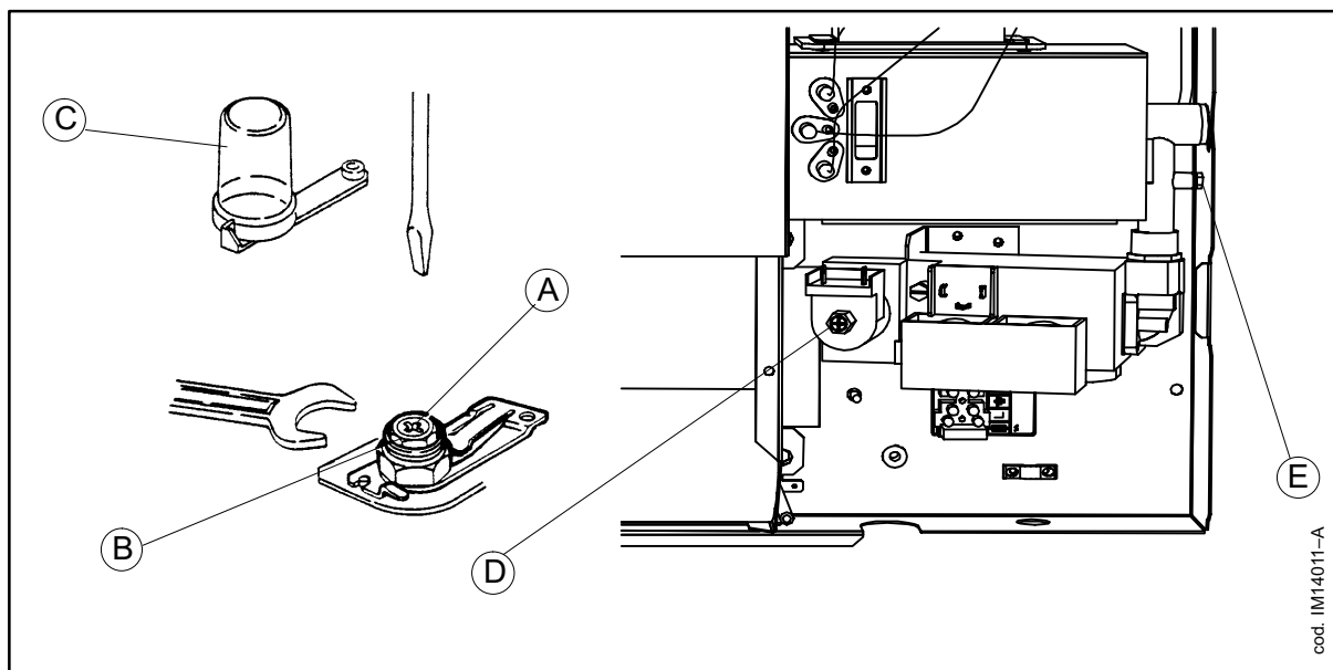
Abb. 27 ELEKTROVENTIL DER MODELLE 5002 U. 8002
