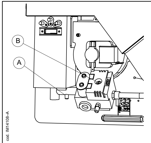
Abb. 26 ELEKTROVENTIL DER GERÄTE 3001 U. 3002
