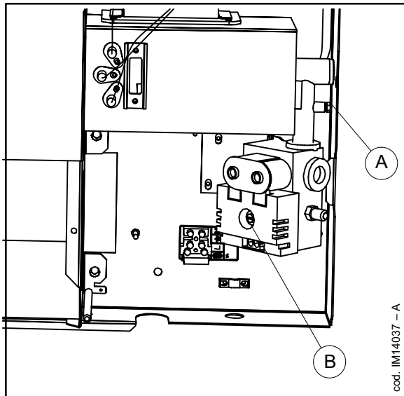
Abb. 25 ELEKTROVENTIL WHITE ROGERS DER MODELLE 4001, 4002 5001 U. 8001
