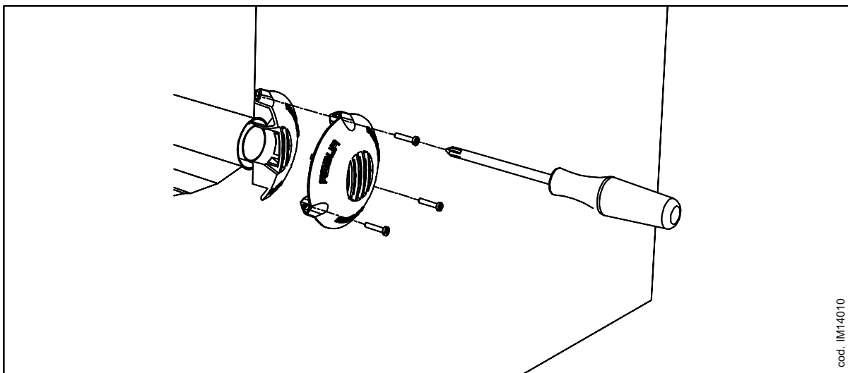
Abb. 24 BEFESTIGUNG DER SCHUTZKAPPE
