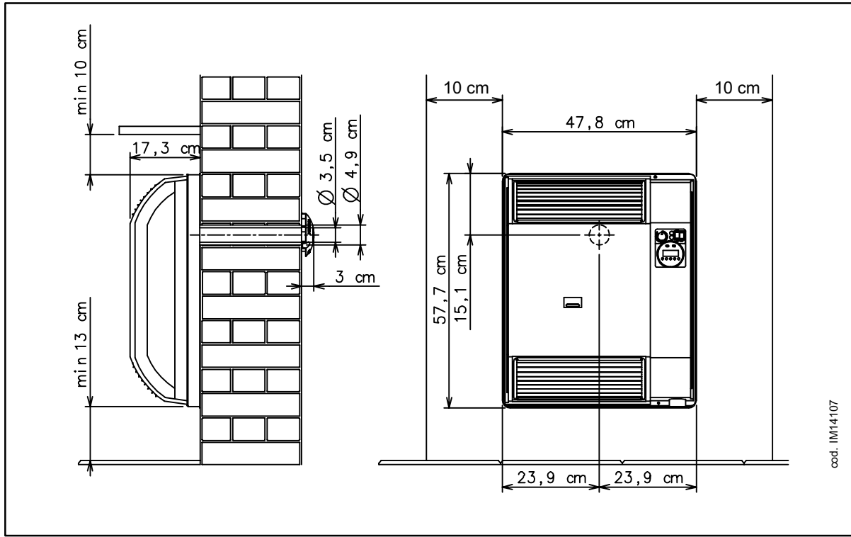
Abb. 1 ÄUSSERE ABMESSUNGEN UND MONTAGERaum FÜR MODELLE 3001-3002
