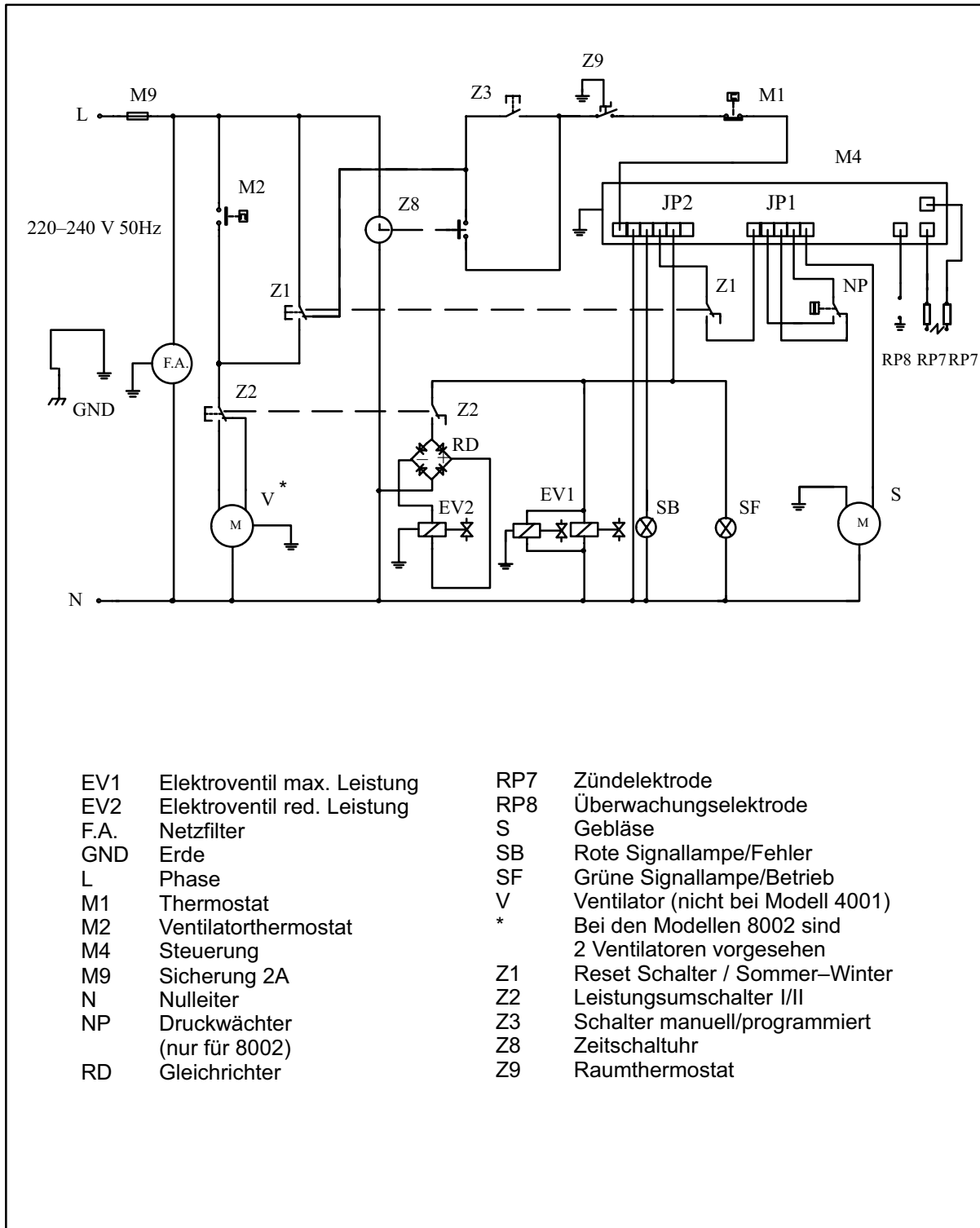
Abb. 32 SCHALTPLÄNE MODELL 5002 U. 8002
