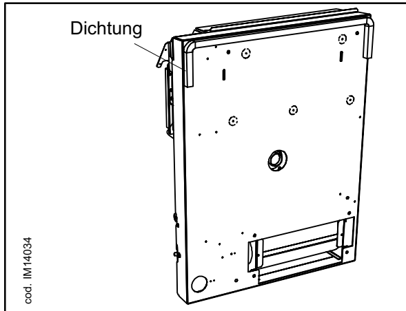
1 Abb. 13 ANBRINGEN DER SELBSTKLEBEDICHTUNG BEI DEN MODELLEN 4001, 4002 , 5001, 5002 8001 U. 8002
