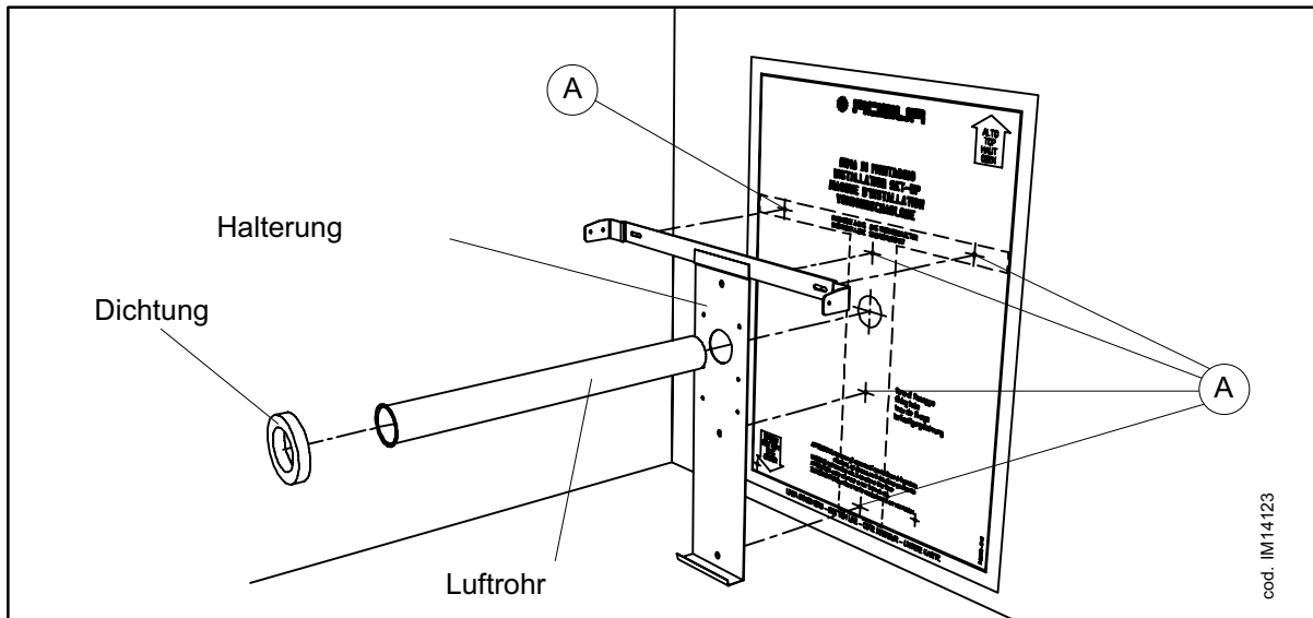
Abb. 8 BEFESTIGUNG DER HALTERUNG UND BOHRUNGEN FÜR DIE MODELLE 4001, 4002, 5001 U. 5002
