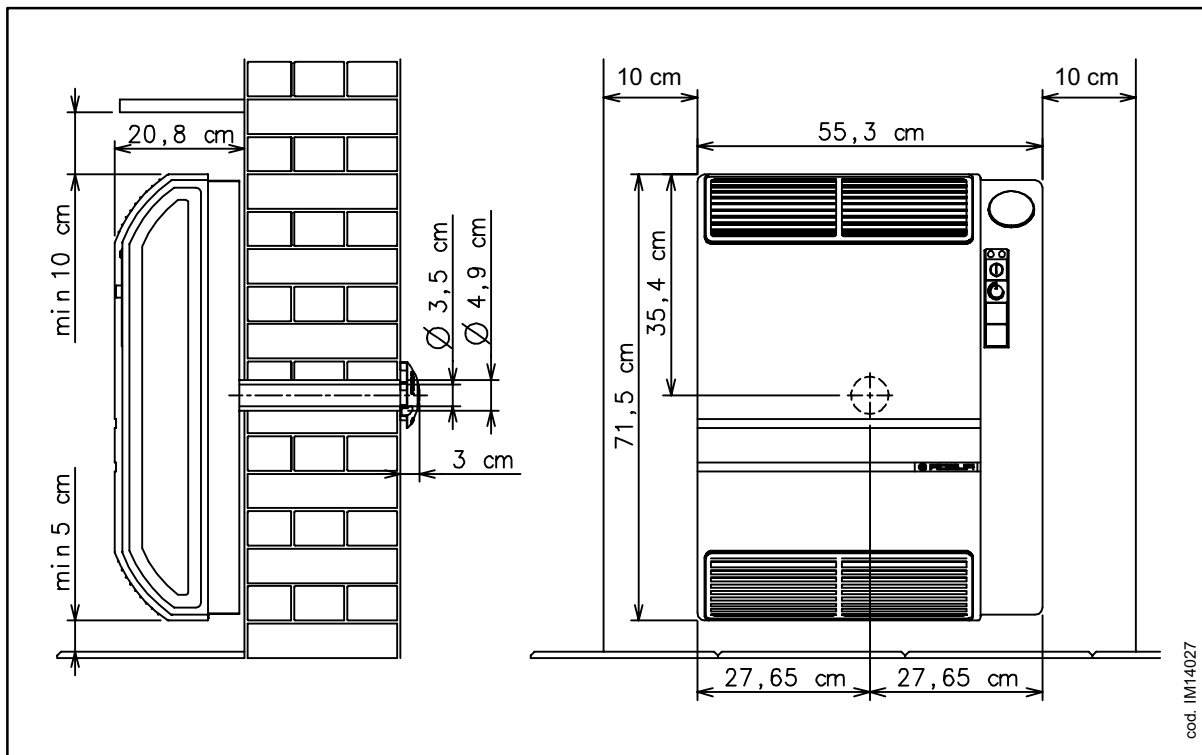
Abb. 2 ÄUSSERE ABMESSUNGEN UND MONTAGERaum FÜR MODELLE 4001-4002-5001-5002
