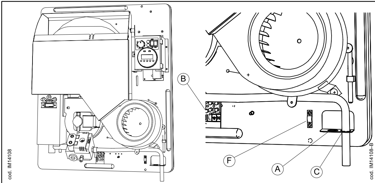
Abb. 23 VERSORGUNGSZUFÜHRUNGEN DER MODELLE 3001 U. 3002
