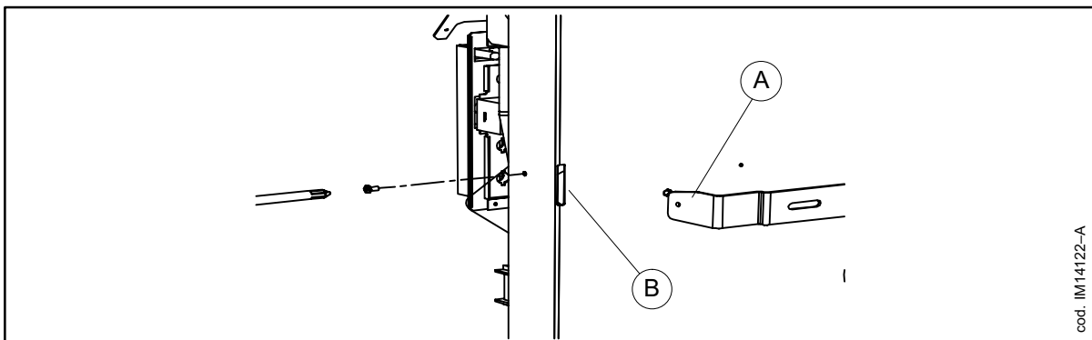
1 Abb. 16 BEFESTIGUNG DER MODELLE 4001, 4002, 5001 U.5002
