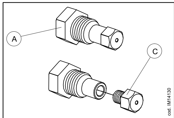
Abb. 30 DÜSENSTOCK MIT DÜSE
