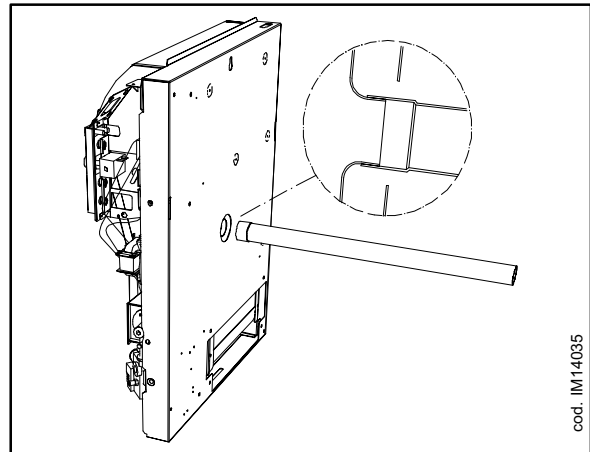
1 Abb. 14 ANBRINGEN DES ABGASROHRES
