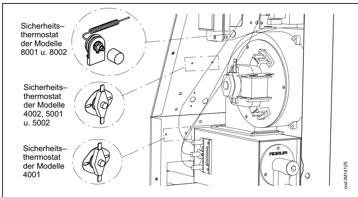
Abb. 36 RESETTASTER SICHERHEITSTHERMOSTAT BEI DEN MODELLEN 4001, 4002, 5001, 5002, 8001 U. 8002
