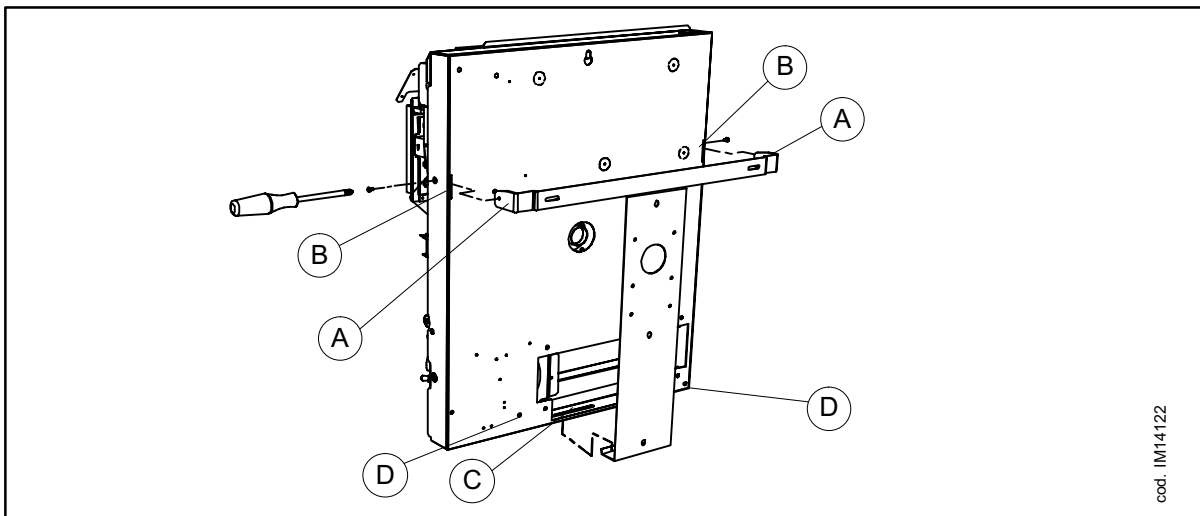
1 Abb. 15 AUFHÄNGUNG DER GERÄTE 4001, 4002, 5001 U. 5002
