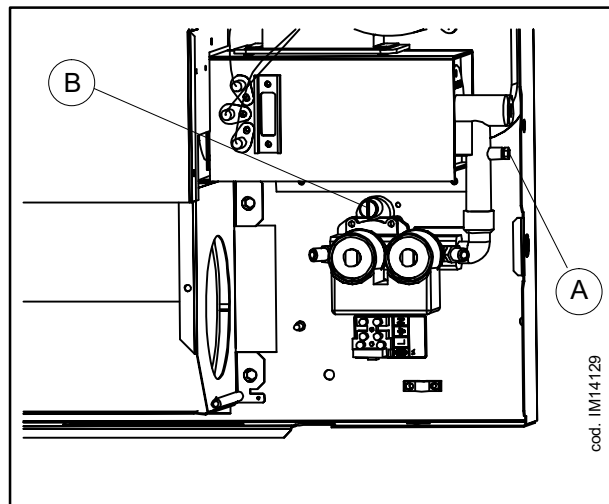
Abb. 28 BRAHMA VENTIL DER MODELLE 4001. 4002, 5001, U. 5002
