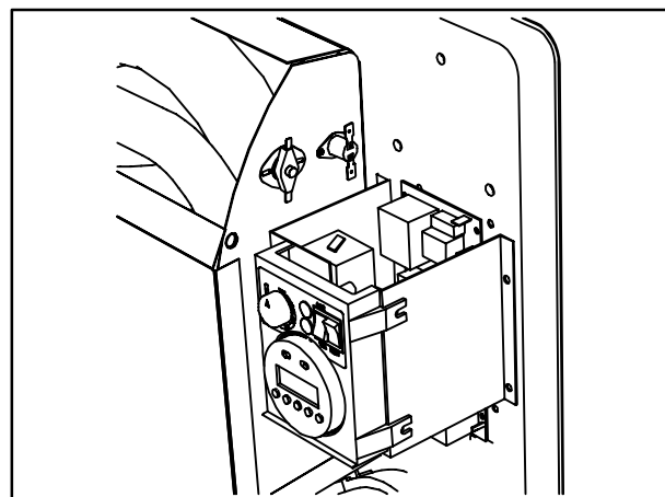
Abb. 37 RESETTASTER SICHERHEITSTHERMOSTAT MODELL 3001 U.3002
