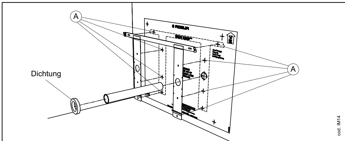
Abb. 9 BEFESTIGUNG DER HALTERUNG UND BOHRUNGEN FÜR DIE MODELLE 8001 U. 8002
