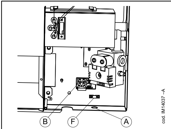
Abb. 21 VERSORGUNGSZUFÜHRUNGEN DER MODELLE 4001, 4002 U. 5001
